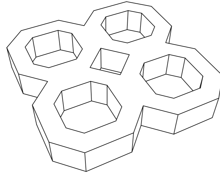
BLOCO INTERTRAVADO VAZADO DIMENSÕES: 50cm x 50cm ESPESSURA: 8cm Pç/m²: 4
