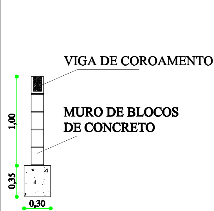
DETALHE CORTE MURO DE BLOCO DE CONCRETO
