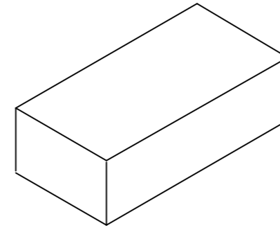
BLOCO INTERTRAVADO DE CONCRETO HOLANDÊS DIMENSÕES: 10cm x 20cm ESPESSURA: 6cm Pç/m²: 50
