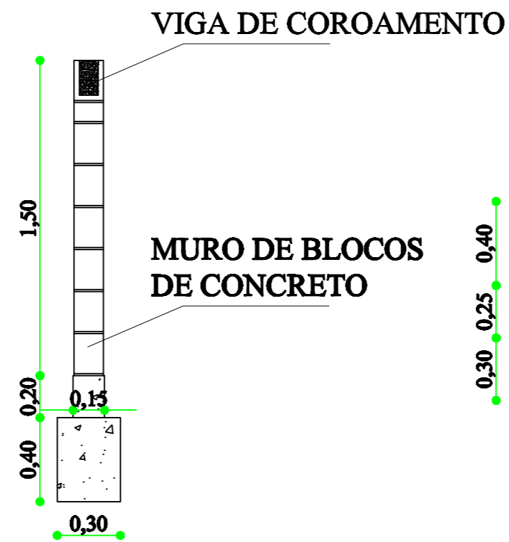
DETALHE CORTE MURO DE BLOCO DE CONCRETO
